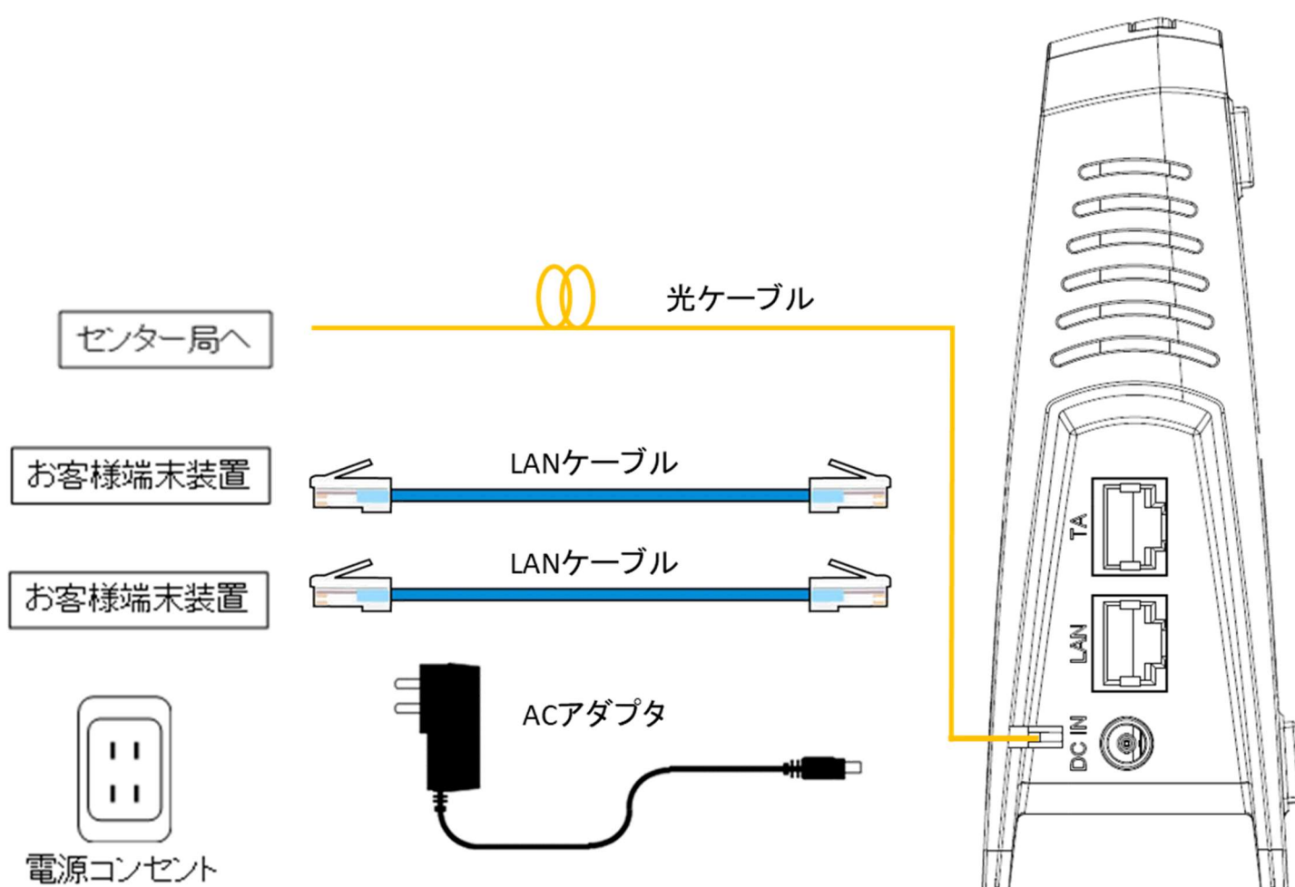
Fig.2 各種ケーブル接続構成図
